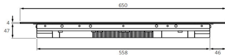
Vue frontale
