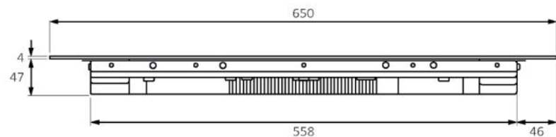
Frontālais skats
