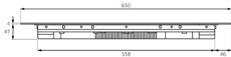
Eestvaade
