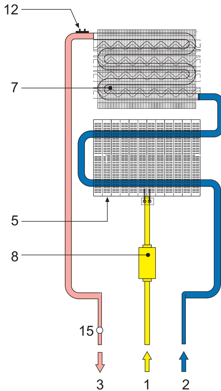
fig. 23 - Circuito idraulico
